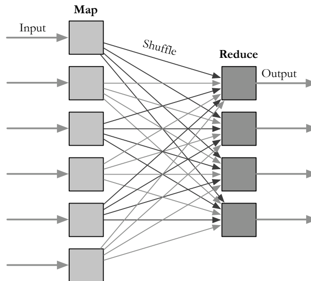
Fig. 5.10. MapReduce
