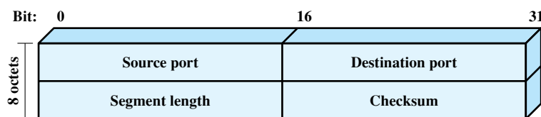
(b) UDP header
